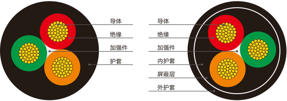
拖链动力电缆结构示意图
