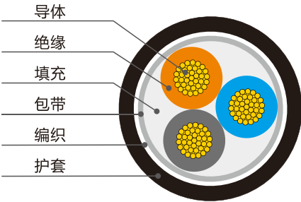
RVVP结构示意图
