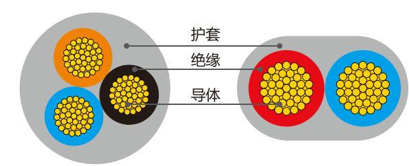
RVV结构示意图
