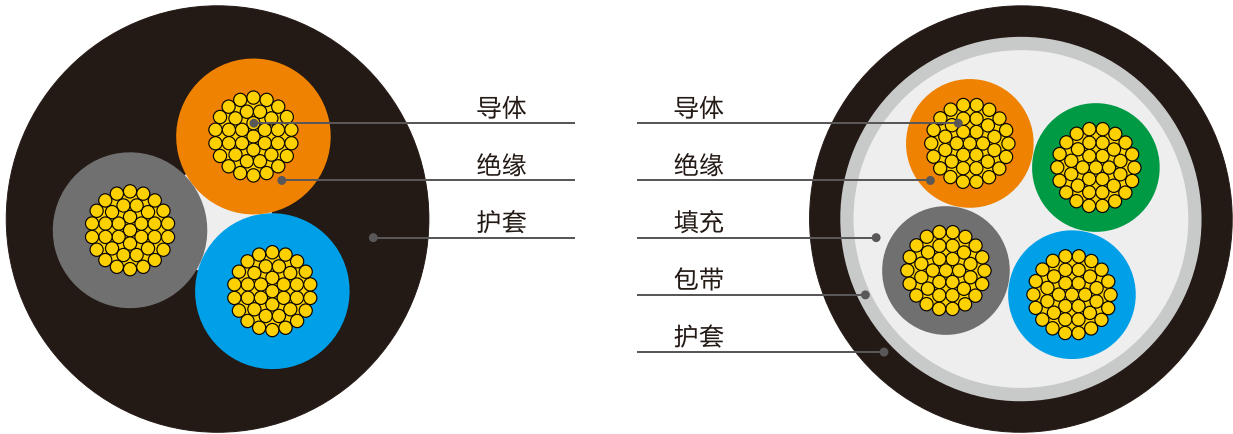
多芯屏蔽（可选）护套线结构示意图
