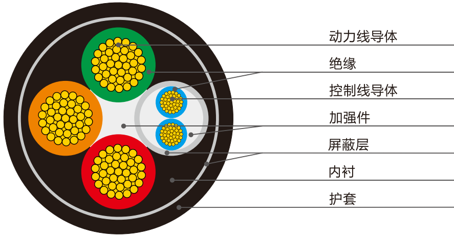
拖链伺服电缆结构示意图
