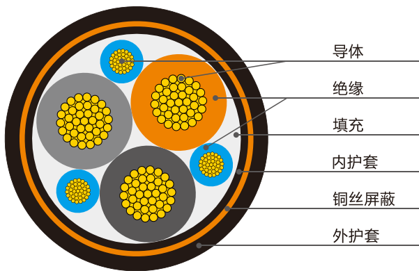
BPYJVP、BPYJYP电缆结构示意图
