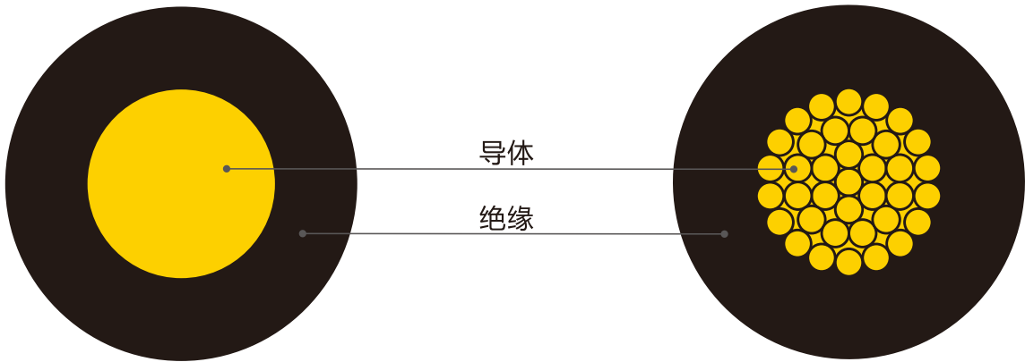
H05V-U、H07V-U结构示意图
