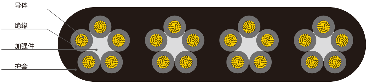
TVVB结构示意图
