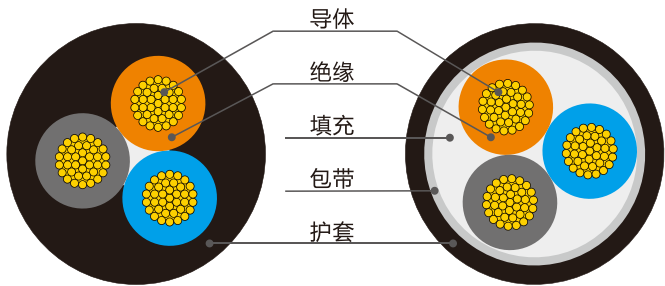
YZ、YZW、YC、YCW结构示意图
