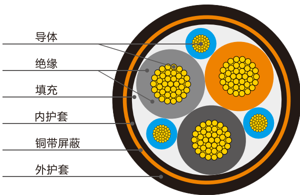
BPYJVP2、BPYJYP2电缆结构示意图
