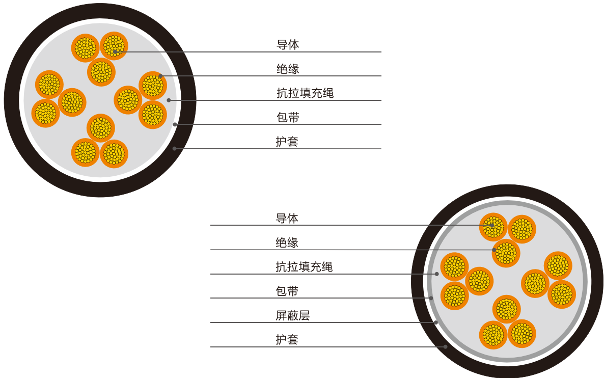
行车控制电缆结构示意图
