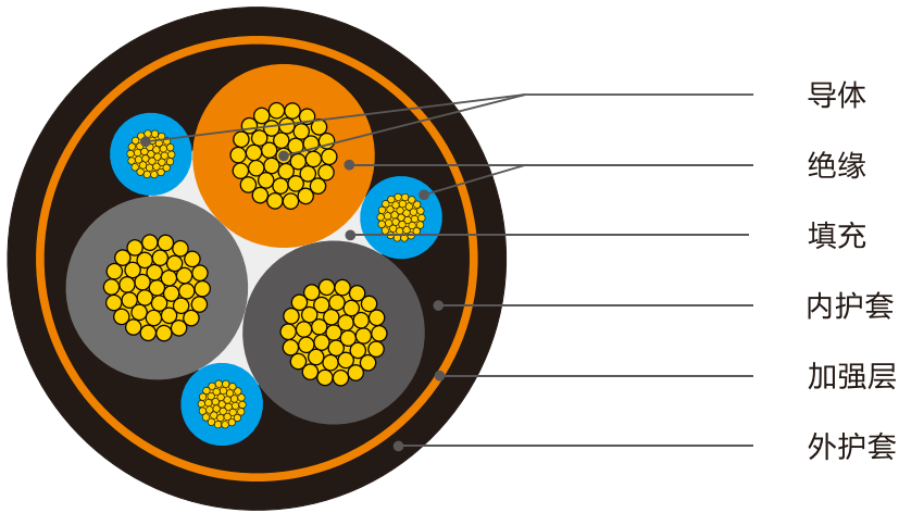
GEUR 起重机专用卷盘电缆结构示意图
