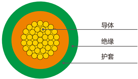
BVV结构示意图
