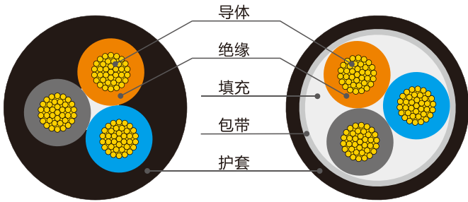
AVVR结构示意图
