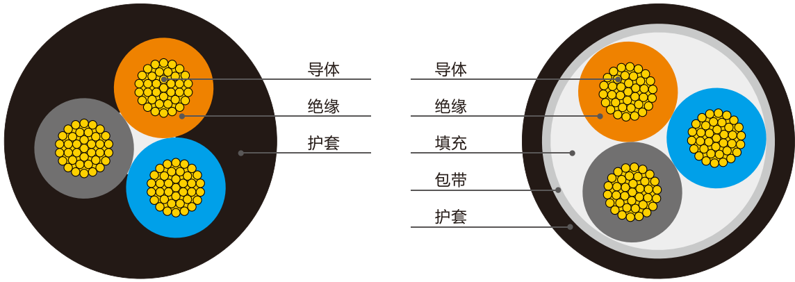
H05VV-F结构示意图
