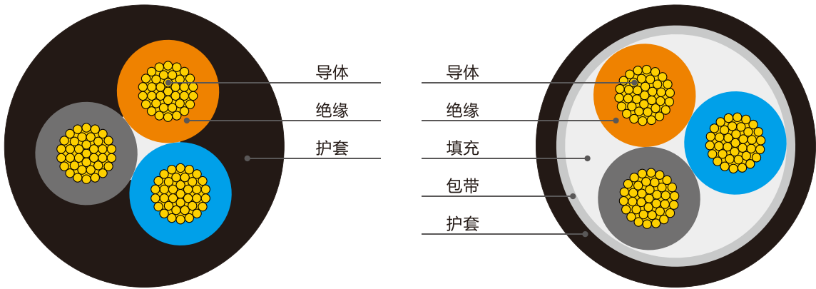
H03VV-F结构示意图
