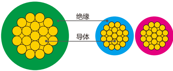
AVR、BV、RV、BVR结构示意图
