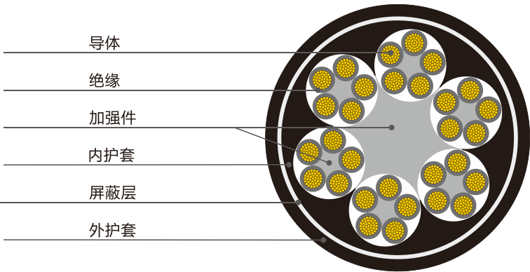
拖链控制电缆结构示意图
