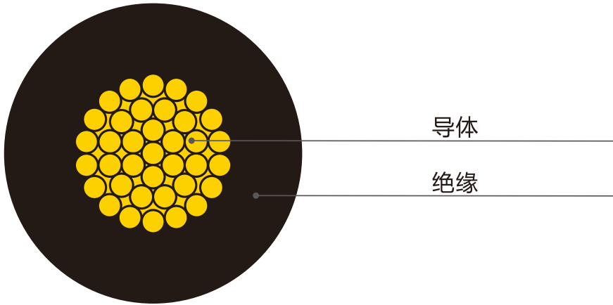
单芯电子连接线结构示意图
