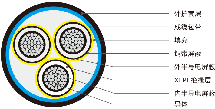
三芯非铠装电缆结构示意图
