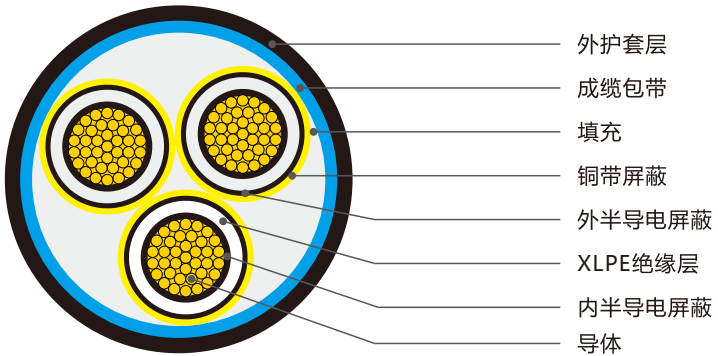
三芯非铠装电缆结构示意图
