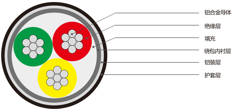
0.6/1KV交联绝缘铠装聚氯乙烯或（低烟无卤）护套铝合金电力电缆结构示意图
