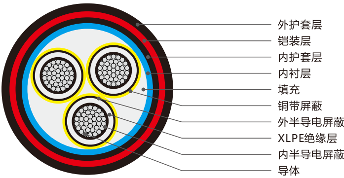
三芯铠装电缆结构示意图
