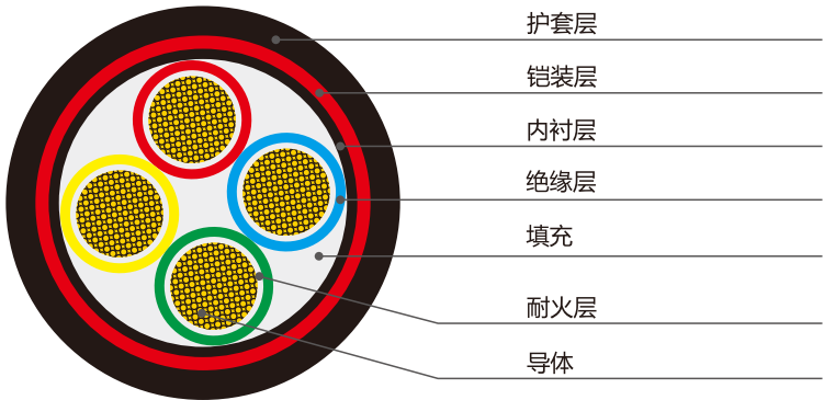
N-VV22 4芯电缆
