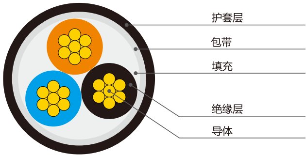
YJV交联电缆结构示意图
