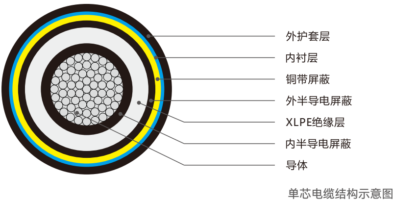
单芯电缆结构示意图
