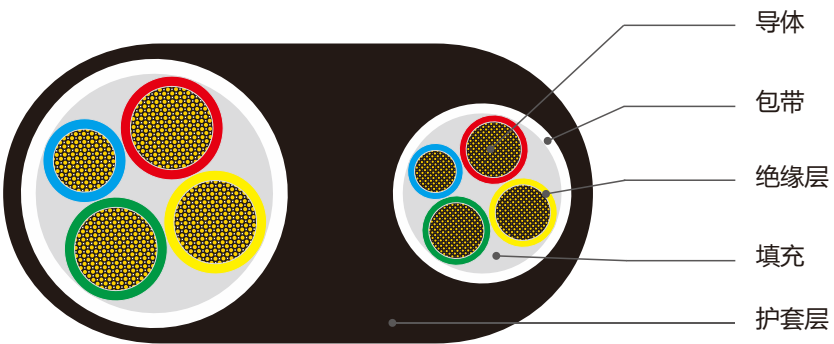
3+1芯预制分支电缆 (FZ-VV、FZ-YJV) 结构示意图
