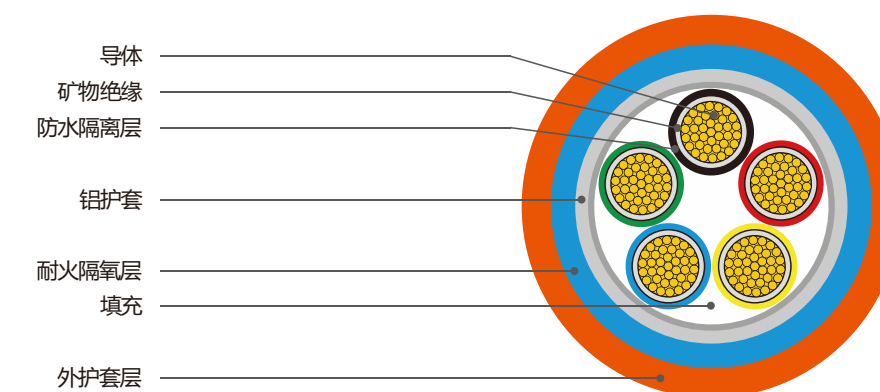
0.6/1kV BTLY 隔离型柔性矿物绝缘铝护套低烟无卤聚烯烃外护套防火电缆结构示意图
