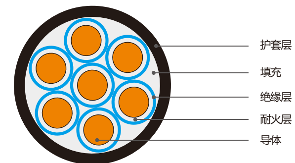
N-KVV结构示意图
