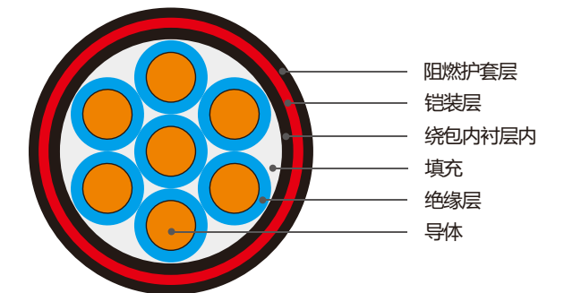
Z (A、B、C) -KVV22及KVV22结构示意图
