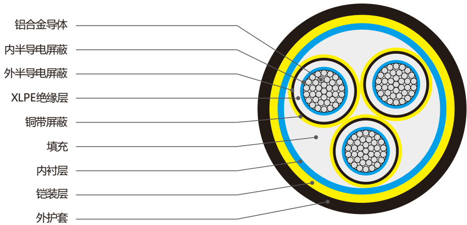
3.6/6KV-26/35KV交联绝缘铠装聚氯乙烯护套铝合金电力电缆结构示意图
