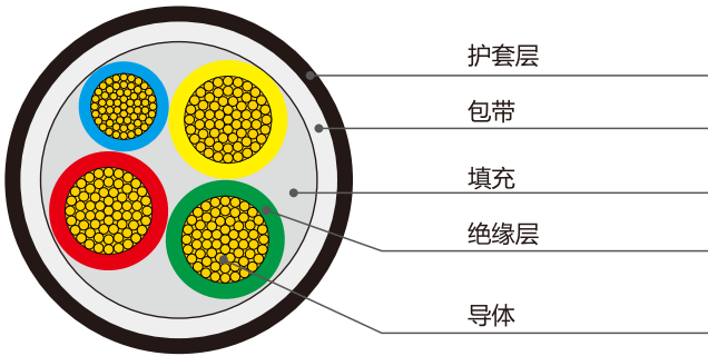
YJV 3+1芯交联电缆结构示意图
