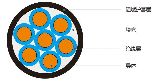
Z (A、B、C) -KVV及KVV结构示意图
