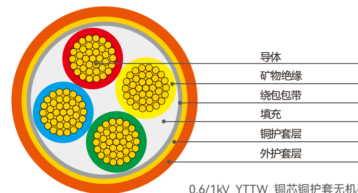
0.6/1kV YTTW 铜芯铜护套无机矿物绝缘电缆结构示意图
