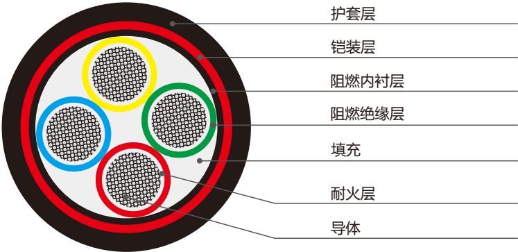
N-VV22 4芯电缆
