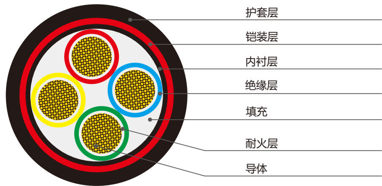
N-VV22 4芯电缆
