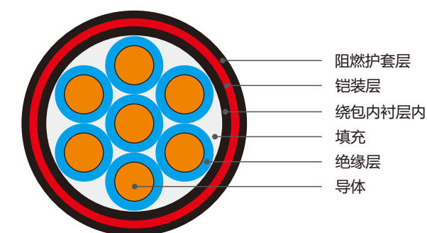
Z ( A、B、C ) -KVV22及KVV22结构示意图
