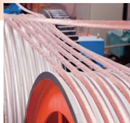
▲ 1+6 (630F) +12高速绞线机
